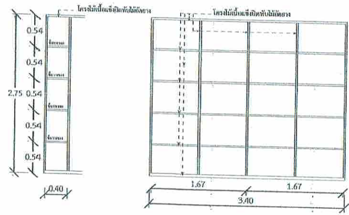
รูปตัดตู้ที่ 3
