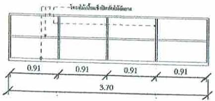
รูปตัดตู้ที่ 1
