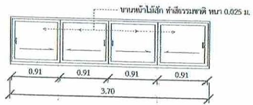
รูปด้านตู้ที่ 1
